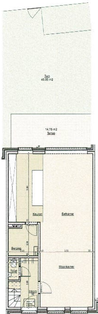
NIVEAU 0
